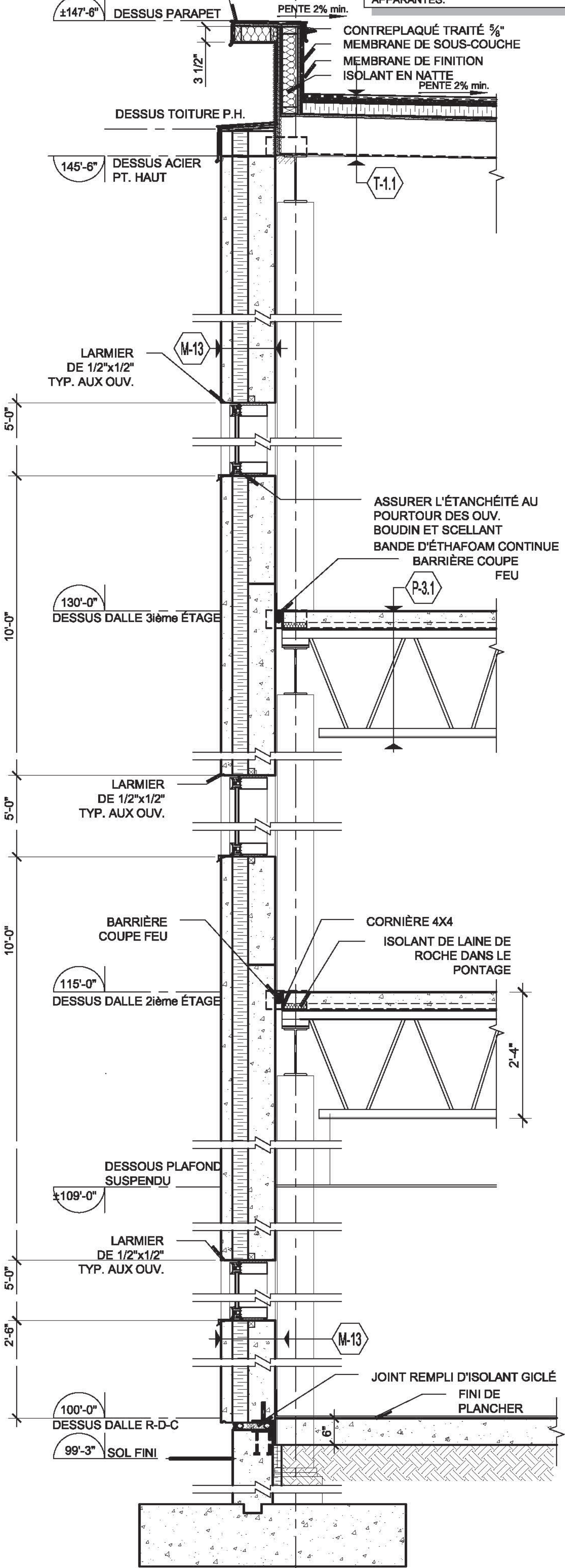
1 COUPE DE MUR - PANNEAU DE BÉTON ÉCHELLE = 1/2" = 1'-0"
